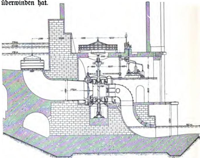
Fig. 70. Beurs Maschinenhaus in Lyon.
